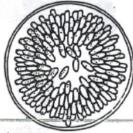
29 Coscinodiscus
